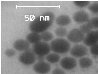
شکل شماره ۴ الف- تصویر میکروسکوپ الکترونی گذار نانو ذرات نقره سنتزی. شرایط: آمونیاک ۰/۷ مولار، فرمالین / نقره کلرید ۲ در غیاب پلی‌وینیل پیرولیدون بعد از یک ماه از سنتز
