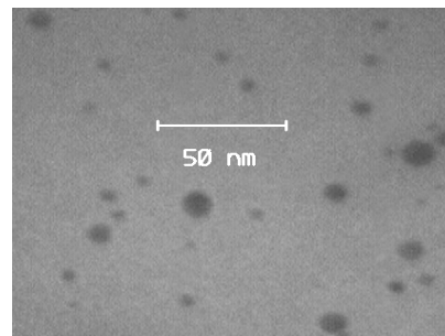
شکل شماره ۳ الف- تصویر میکروسکوپ الکترونی گذار از نانو ذرات نقره سنتزی. شرایط سنتز: آمونیاک ۰/۷ مولار، فرمالین / نقره کلرید ۲ در حضور پلی‌وینیل پیرولیدون بعد از یک ماه از سنتز
