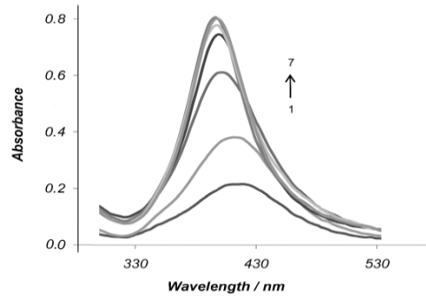
شکل شماره ۲ الف- تاثیر نسبت مولی فرمالین به نقره کلرید بر طیف پلاسمون نانوقره در حضور ۰/۷ مولار از آمونیاک (۱) ۰/۱ (۲) ۰/۵ (۳) ۱/۰ (۴) ۱/۵ (۵) ۲/۰ (۶) ۲/۵ (۷) ۳/۰
