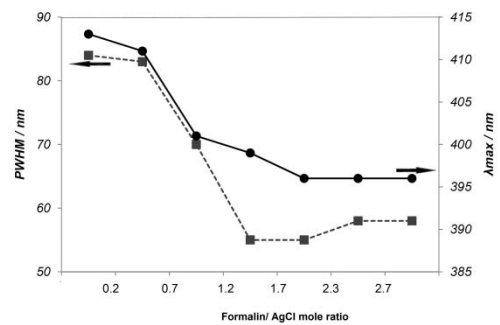
شکل شماره ۲ ب- تاثیر نسبت مولی فرمالین به نقره کلرید بر پهنای پیک در نصف ارتفاع و طول موج ماکزیمم جذب در غلظت ۰/۷ مولار از آمونیاک
