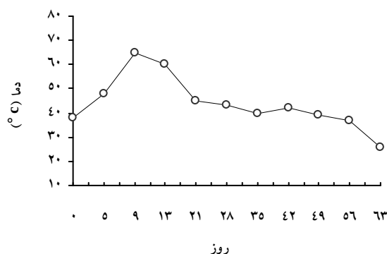
نمودار شماره ۱- تغییرات دمای توده کمپوست در طی فرایند کمپوست
