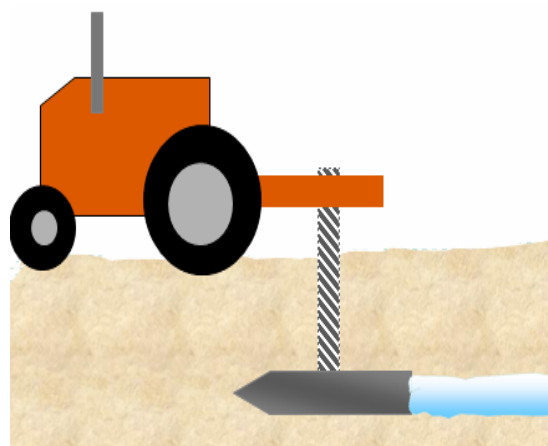
شکل شماره ۴- زهکشی به‌طریقه مول (شکل از ر. دهقانی)
