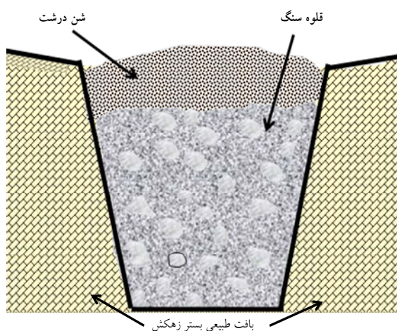
شکل شماره ۱- برش عرضی یک زهکش ساده‌ی زیر زمینی: جوی زیر زمینی که با لایه‌هایی از قلوه سنگ پر شده و سپس روی آن با شن درشت پوشانده شده است (شکل از ر. دهقانی)
