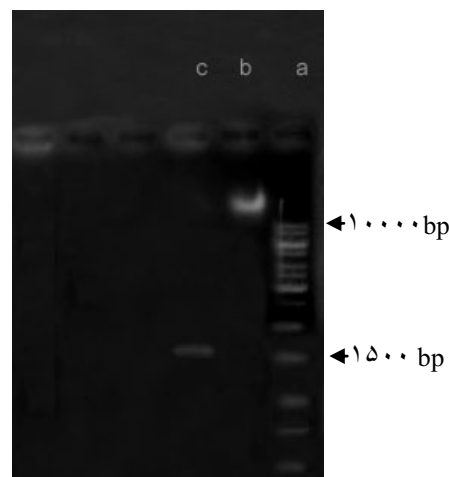
شکل شماره ۲- باند مربوط به DNA استخراج شده از باکتری نمک دوست نسبی مقاوم به نیکل Salinivibrio costicola و محصول تکثیر ژن 16S rDNA آن به روش PCR با استفاده از آغازگرهای 27F و 1492R (a) نشان گر ۱ کیلو بازی، b: باند حاصل از DNA استخراج شده، c: باند محصول تکثیر ژن 16S rDNA .
