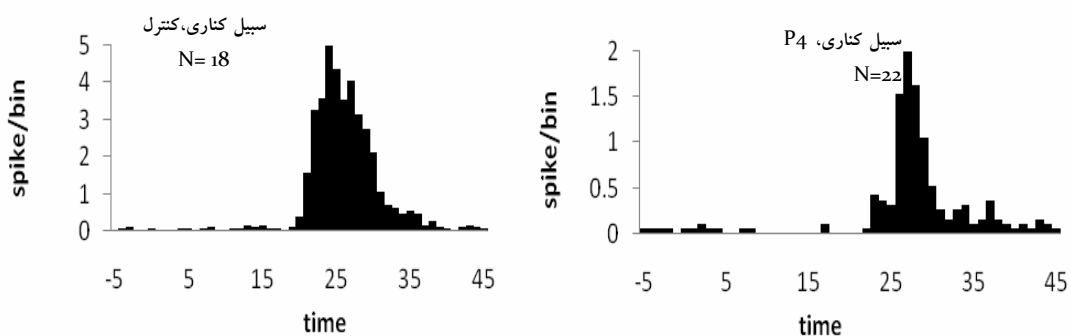
شکل شماره ۳ - مقایسه هیستوگرام تجمعی پاسخ نوروها بعد از تحریک ویسکر کناری در گروه های کنترل و گروه P4. هر هیستوگرام تجمعی نشان دهنده پاسخ نوروها به ۴۰ بار تحریک ویسکر کناری است. محور افقی نشان دهنده زمان برحسب میلی ثانیه است و زمان صفر، نشان گر لحظه شروع تحریک ویسکر است. محور عمودی در هر دو نمودار مشابه و بر حسب Spike/Bin است
