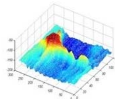
نمودار شماره ۳- نمودارهای مربوط به حفره ایجاد شده با تابش ۸۰۰ پالس و انرژی ۷۰ میلی ژول از لیزر زنون کلراید روی بافت عاج
