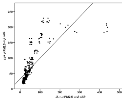
نمودار شماره ۱- رابطه بین غلظت ذرات PM_{2.5} ( \mu\text{g m}^{-3} ) در هوای داخل و خارج بیمارستان نقوی شهر کاشان
