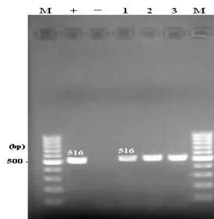
شکل شماره ۱- الکتروفورز ژل آگارز. M: مارکر ۱۰۰ جفت بازی؛ ستون +: کنترل مثبت برای ژن qnrA (اشریشیا کلی حامل qnrA )؛ ستون -: کنترل منفی، شامل مخلوط واکنش PCR با افزایش آب دیونیزه به جای DNA الگو؛ ستون‌های ۱-۳: جدایه‌های بالینی مثبت از نظر ژن qnrA
