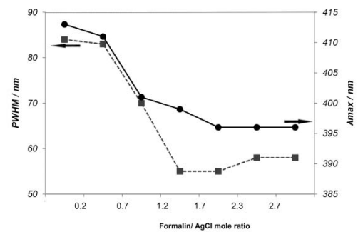
شکل شماره ۲ ب) تاثیر نسبت مولی فرمالین به نقره کلرید بر پهنایی پیک در نصف ارتفاع و طول موج ماکزیمم جذب در غلظت ۰/۷ مولار از آمونیاک
