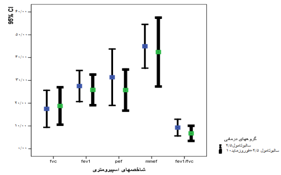
نمودار شماره ۱- میانگین و فاصله اطمینان ۹۵ درصد برای درصد تغییر شاخص‌های اسپیرومتري گروه‌های درمانی سالیوتامول با و بدون فوروزماید بعد از درمان
