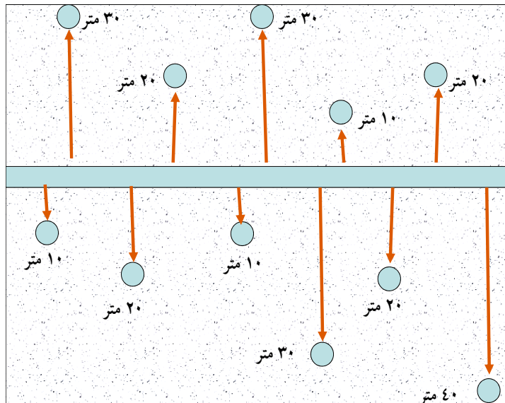
شکل شماره ۱۴- نحوه تعیین فواصل زهکش‌های فرعی (شکل از ر. دهقانی)
