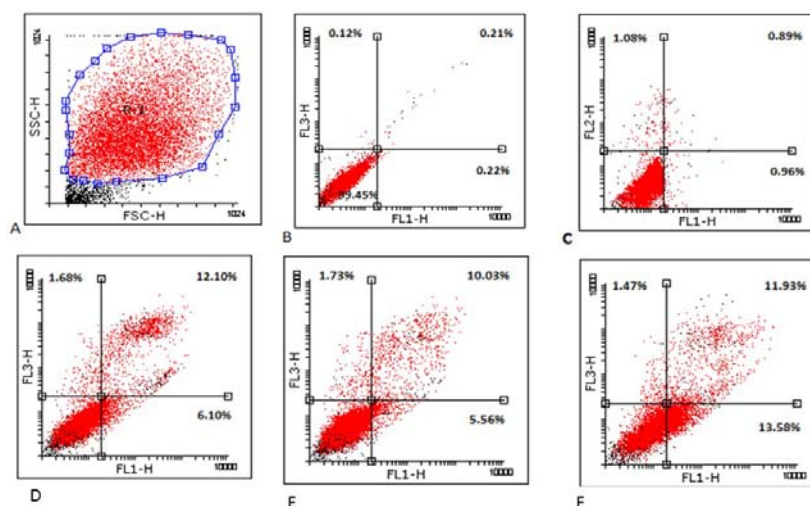
شکل شماره ۳- مقایسه‌ی بیان انکسین و پروپیدیم بدید در نمونه‌های تیمار شده و نشده با کوئرستین و عصاره پوست انار با استفاده از روش فلوسایتمتری. در هر کدام از نمودارها آن دسته از سلول‌هایی که در بخش پایین - چپ قرار دارند، سلول‌های کامل سالم را نشان می‌دهند. سلول‌های بخش بالا - چپ سلول‌های دچار نکروز، بخش بالا راست سلول‌های مرحله Late Apoptosis و بخش پایین راست سلول‌هایی را که در مرحله Early Apoptosis قرار دارند، را نشان می‌دهند. شکل (A) برای تنظیم دستگاه، (B) گروه رنگ‌نشده، (C) گروه تیمار نشده، (D) گروه تیمار شده با 1\mu\text{M} کوئرستین، (E) گروه تیمار شده با 100\mu\text{g/ml} عصاره پوست انار، (F) گروه تیمار شده با کوئرستین و عصاره پوست انار به‌طور هم‌زمان.
