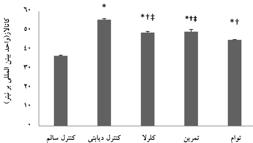
نمودار شماره ۲- مقدار کاتالاز در مغز موش‌های گروه‌های مورد بررسی پس از اعمال مداخله داده‌ها به صورت میانگین و انحراف معیار گزارش شده‌اند ( N=10 ). *، †، ‡: به ترتیب نمایانگر تفاوت معنی‌دار نسبت به گروه کنترل سالم، کنترل دیابتی و توام ( P < 0.05 ) بر اساس نتایج آزمون تعقیبی توکی.
