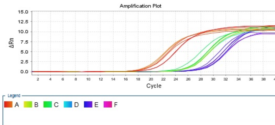
شکل شماره ۴- نمودار تکثیر ژن‌های مورد مطالعه Bax ، Bcl2 و \beta -actin همانطور که مشاهده می‌شود از سیکل ۱۸ به بعد میزان فلورئوسانس نمونه افزایش می‌یابد که نشان‌دهنده تکثیر ژن‌های مدنظر است. رنگ قرمز ژن Bax ، رنگ سبز ژن Bcl2 و رنگ آبی ژن \beta -actin بود.
