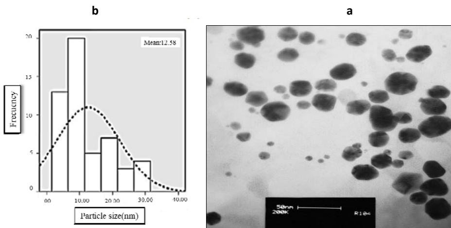
شکل شماره ۱- تصویر حاصل از عکس‌برداری از نانوذرات نقره با استفاده از میکروسکوپ الکترونی گذاره، b- نمودار حاصل از اندازه‌گیری نانوذرات نقره
