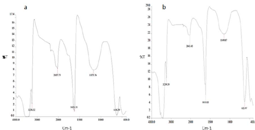
شکل شماره ۲- نمودار حاصل از طیف‌سنجی مادون قرمز. در این تصویر نمودار a نشان دهنده طیف عصاره گیاه بومادران به‌تنهایی می‌باشد، درحالی‌که نمودار b طیف حاصل از نانوذرات نقره را نشان می‌دهد. شباهت دو طیف تایید پوشش سطحی نانوذرات از جنس عصاره گیاهی می‌باشد.
