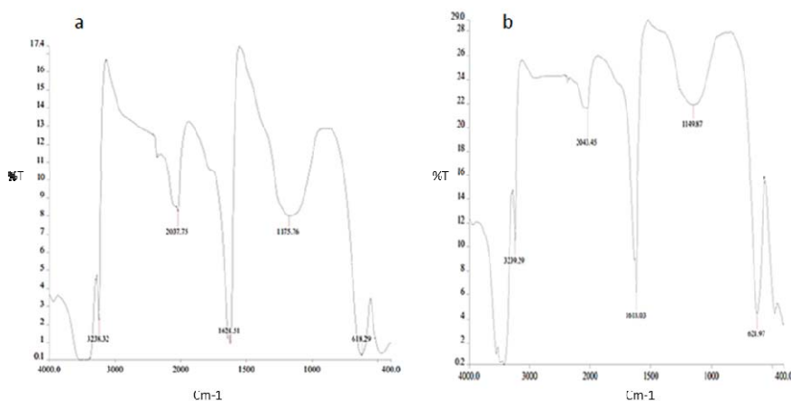
شکل شماره ۲- نمودار حاصل از طیف‌سنجی مادون قرمز. در این تصویر نمودار a نشان دهنده طیف عصاره گیاه بومادران به‌تنهایی می‌باشد، در حالی که نمودار b طیف حاصل از نانوذرات نقره را نشان می‌دهد. شباهت دو طیف تایید پوشش سطحی نانوذرات از جنس عصاره گیاهی می‌باشد.
